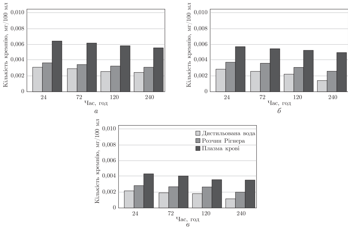
Рис. 2. Інтенсивність розчинення кремнію в дистильованій воді, розчині Рінгера та плазмі крові людини для порошкової системи ГАП + 10% БЛ за різних умов температурного режиму обробки: a – 700 °С, б – 900 °С, в – 1200 °С
